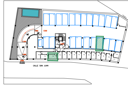
PLANTA SÓTANO
