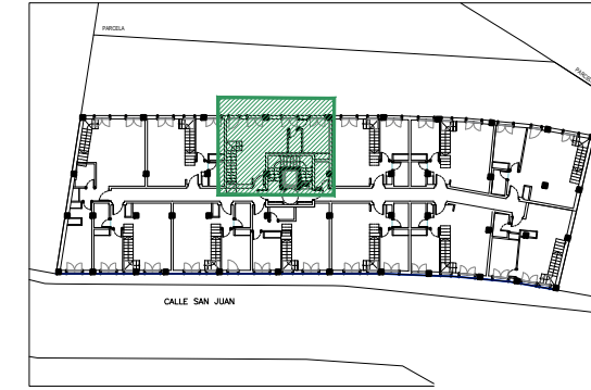
PLANTA PRIMERA
